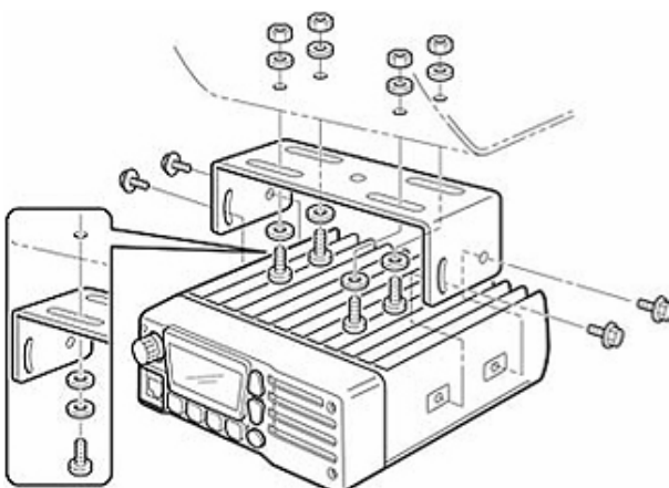
Крепежный комплект FL-M1000E/A
