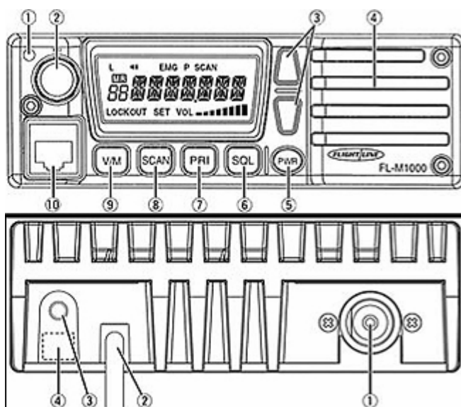
Органы управления FL-M1000E/A
